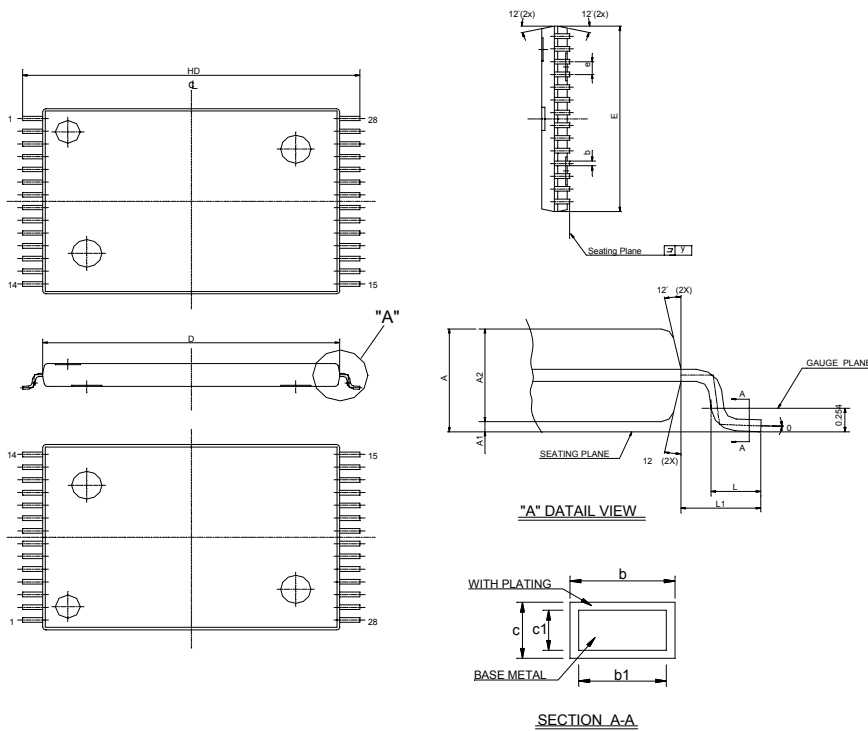
TSOP - 28
