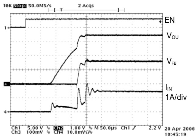
Start Up 700mA Flash V_{IN}=3.6V , V_{OUT}=3.6V
