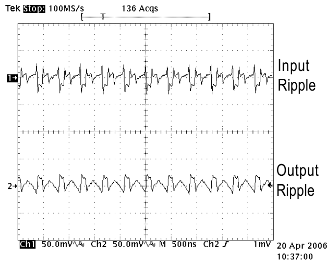
Ripple 2X Flash 700mA, V_{IN}=3.6V
