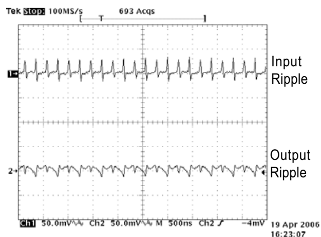
Ripple 2X Flash 1000mA, V_{IN}=3.6V
