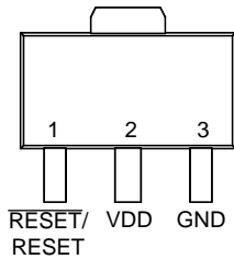
SOT-89
