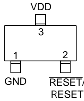
SC-70-3
