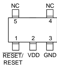
SOT-23-5
