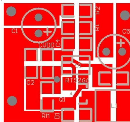
- Top Layer -
