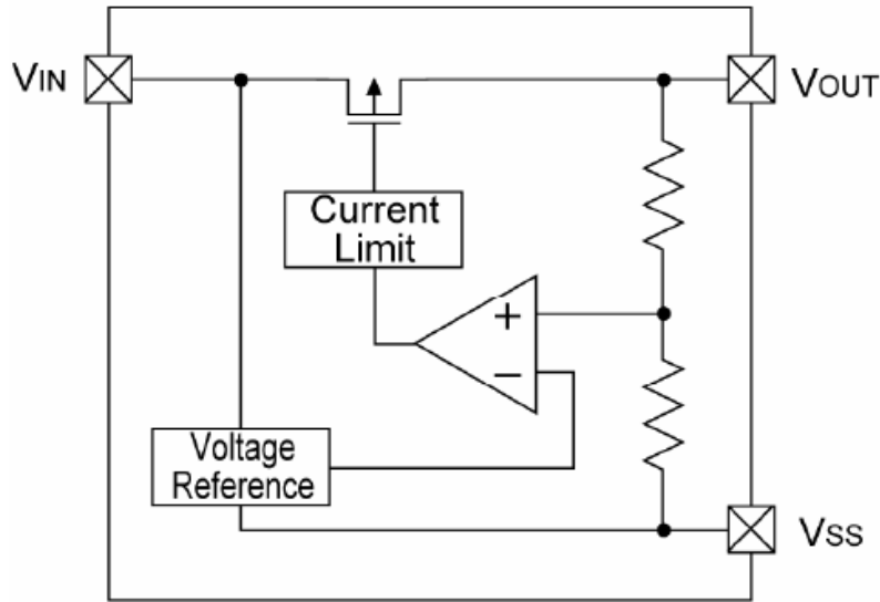
Circuit 2 :
