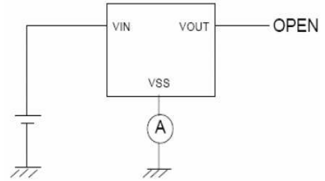
Circuit 2 :
