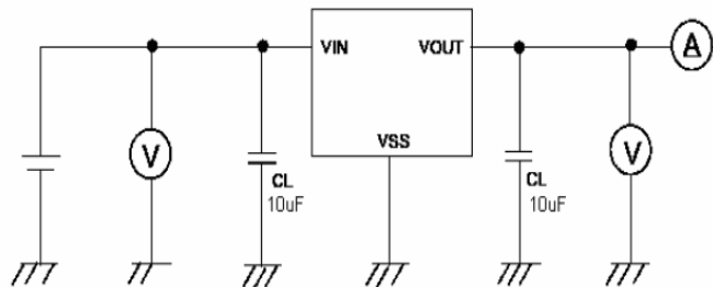
Circuit 1 :
