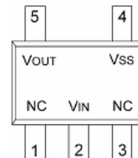
SOT-353
