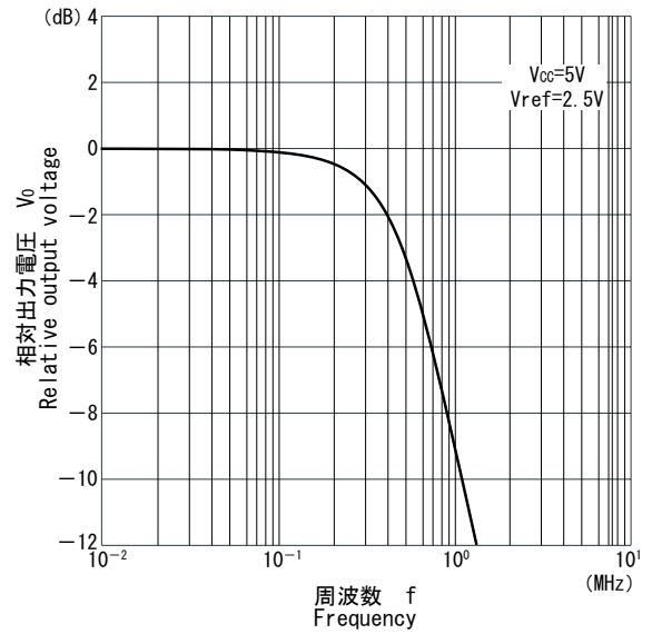
■周波数特性 Tracking
