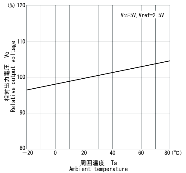
■出力電圧/周囲温度特性 V_o/T_a
