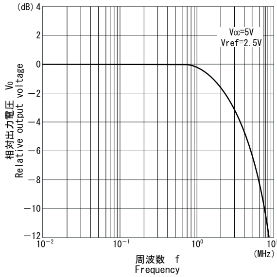
■周波数特性 Focus
