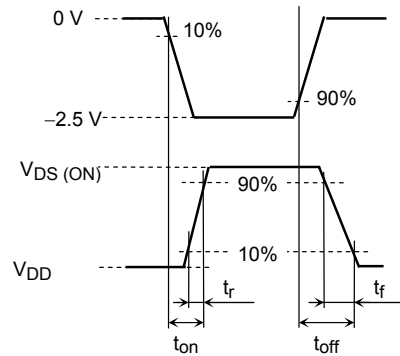
(c) 出力波形
