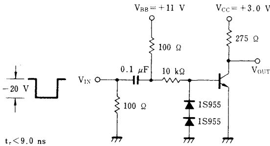
t off 測定回路
