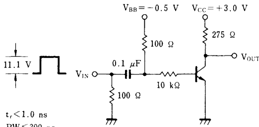
t on 測定回路
