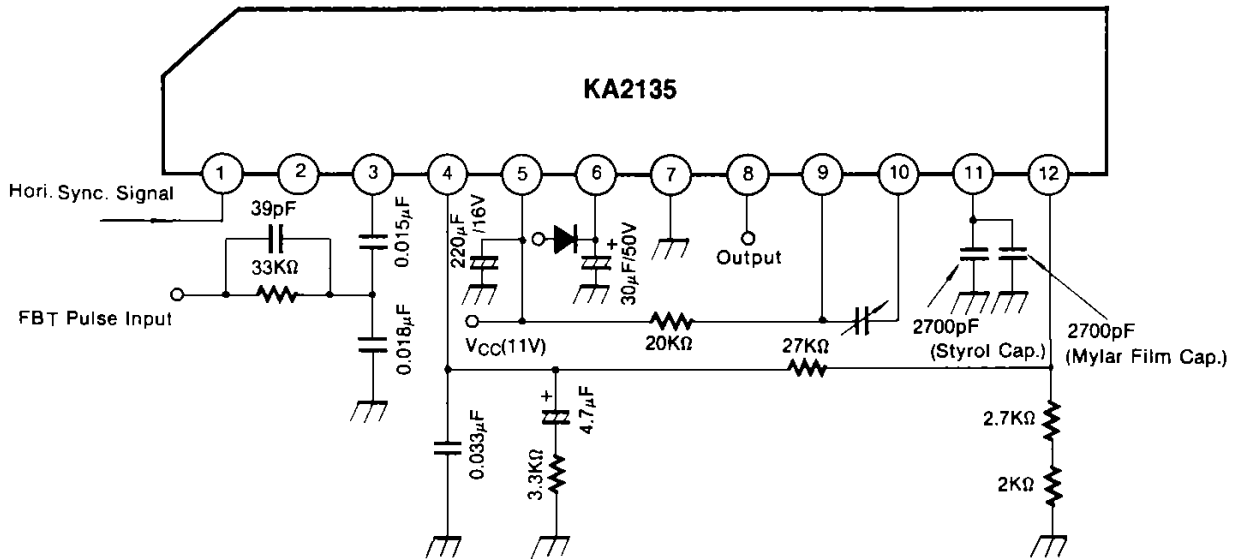
Test Circuit 1 (V 2,7 )
