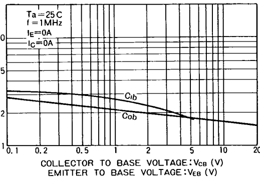
Fig.10 入出力容量—電圧特性
