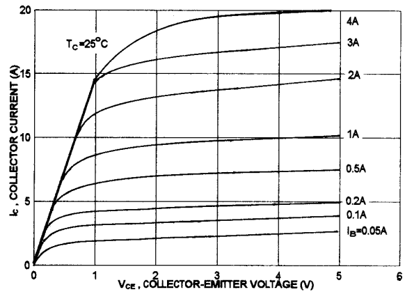
IC - Vce
