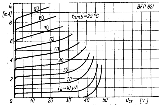
Charakterystyka wyjściowa I_C = f(U_{CE}) ; I_B — parametr
