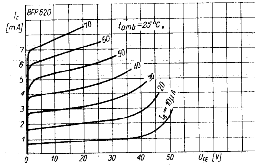
Charakterystyka wyjściowa I_C = f(U_{CE}) ; I_B — parametr
