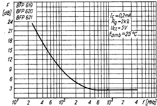
Zależność współczynnika szumów od częstotliwości F = f(f)
