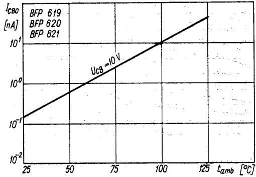
Zależność temperaturowa prądu zerowego I_{CB0} = f(t_{amb})
