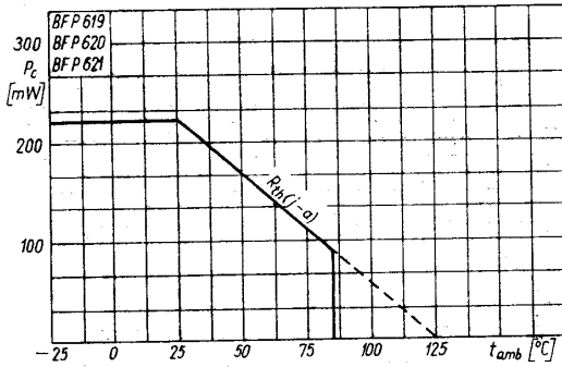
Zależność temperaturowa mocy strat P_C = f(t_{amb})
