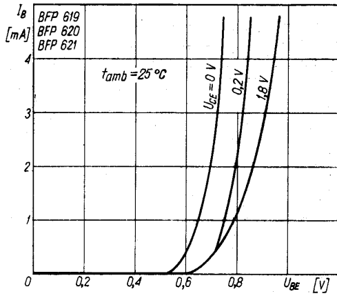
Charakterystyka wejściowa I_B = f(U_{BE})
