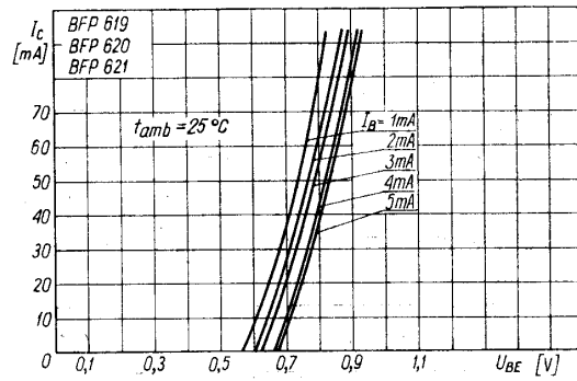
Charakterystyka przejściowa I_C = f(U_{BE})
