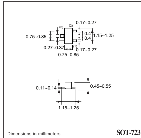
SOT-723
