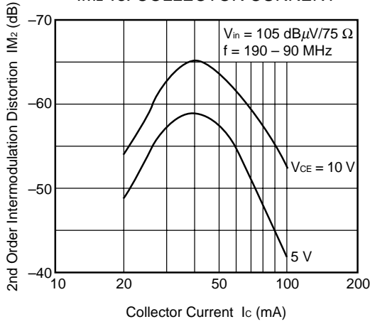
IM 2 vs. COLLECTOR CURRENT
