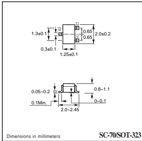
SC-70/SOT-323
