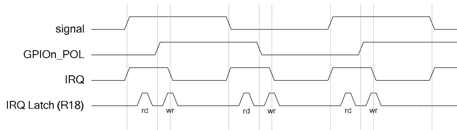
Figure 27 GPIO Edge Detect
