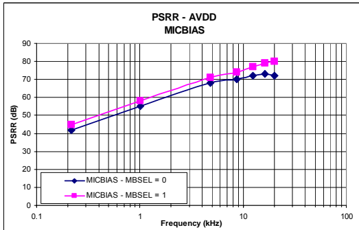
AVDD – MICBIAS
