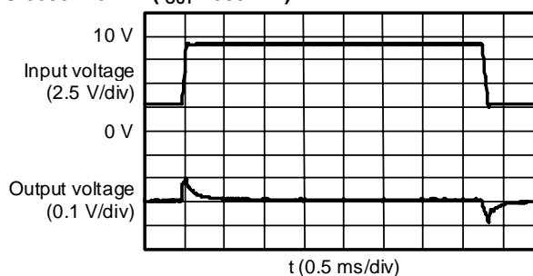
S-8533A33AFT ( I_{OUT} : 500\text{ mA} )
