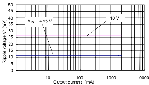
(33) S-8533A50AFT (CPH6302/CPH6402)
