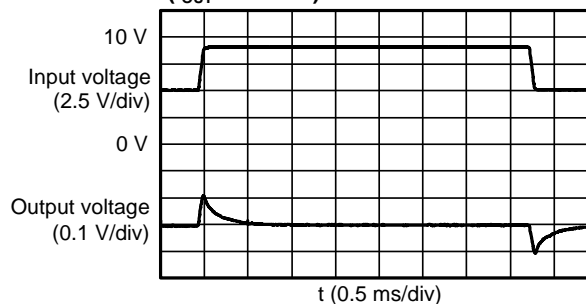
S-8533A50AFT ( I_{OUT} : 500\text{ mA} )
