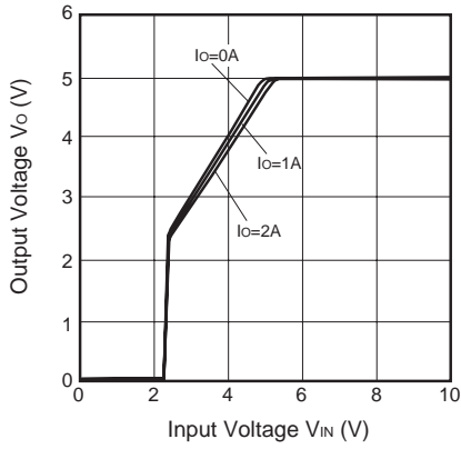
Fig.9 Output Voltage vs. Input Voltage (PQ050RDA2SZH)
