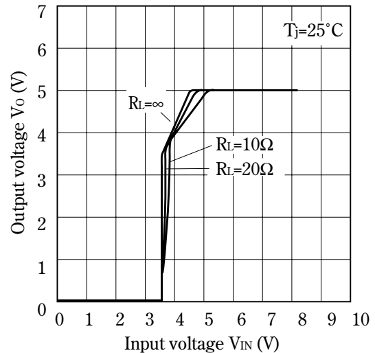
Fig.9 Output Voltage vs. Input Voltage (PQ05SZ5/PQ05SZ51)
