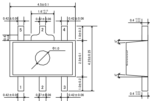
SOT-89-5
