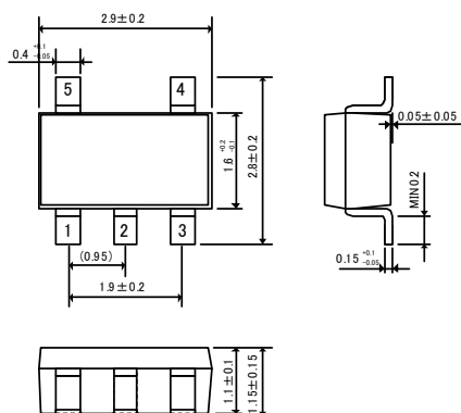
SOT-25
