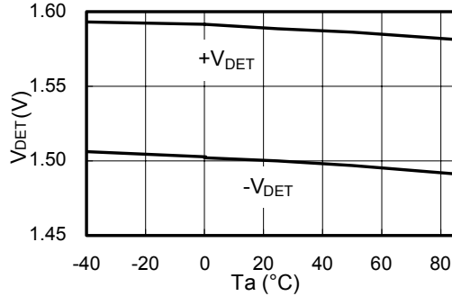
S-80815CL
