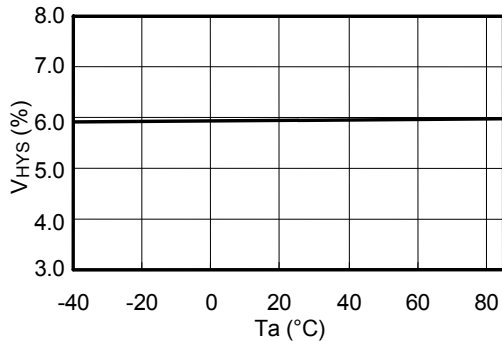
S-80815CL
