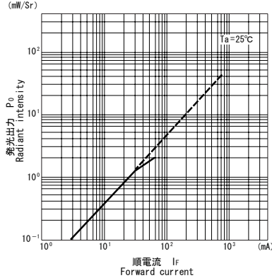
■発光出力／順電流特性 P_0/I_f
