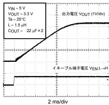
起動特性 ( C_{SS} = 0.1\mu F )
