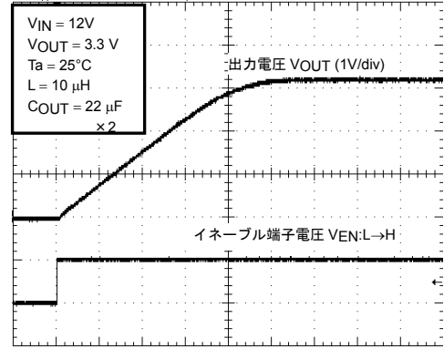
起動特性 ( C_{SS} = 0.1\mu\text{F} )
