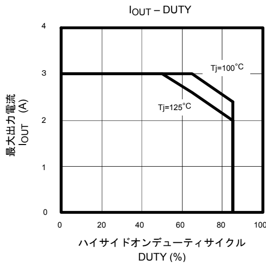
図 6 安全動作領域
