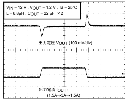
負荷応答特性
