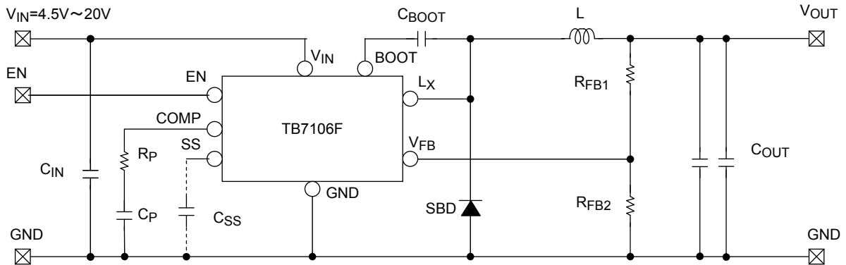
図 1 TB7106F 応用回路例
