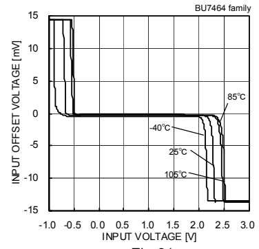
Fig. 61 Input Offset Voltage – Input Voltage (VDD=3[V])
