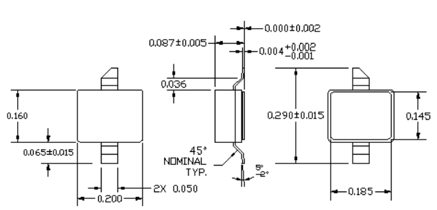
POLYFET S02 PACKAGE
