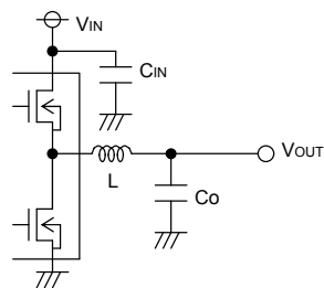
Input Capacitor
