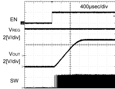
Fig.13 EN wake up
