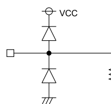
12pin (Is-)
