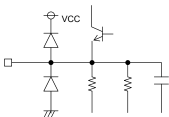
7pin (VREG)
