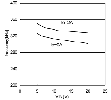
Fig.9 VIN vs f
