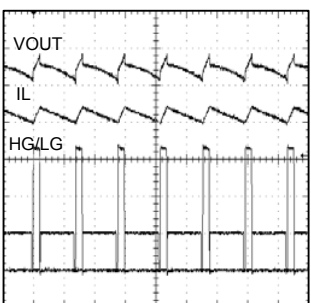
Fig.21 SLLM Mode (IOUT=1A)
