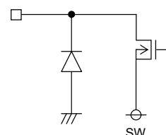
39pin (EN)
