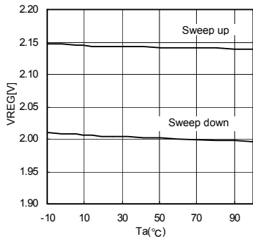
Fig.4 Ta vs UVLO (VREG)
