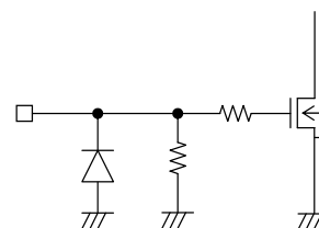
39pin (EN)
