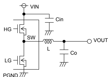
Input Capacitor
