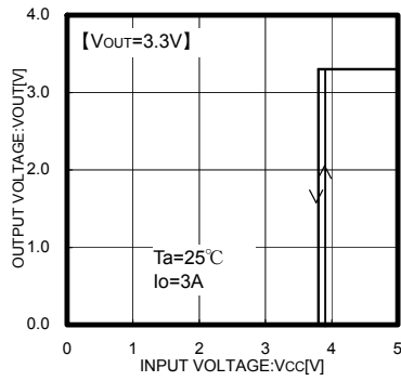
Fig.3 Vcc - VOUT
