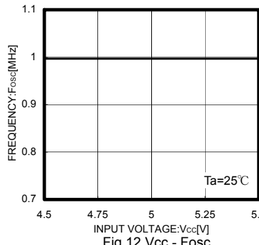
Fig.12 Vcc - Fosc
