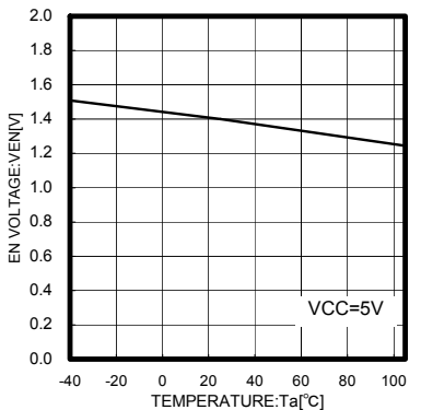
Fig.10 Ta - VEN
