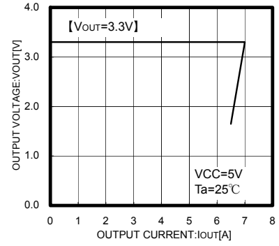
Fig.5 IOUT - VOUT
