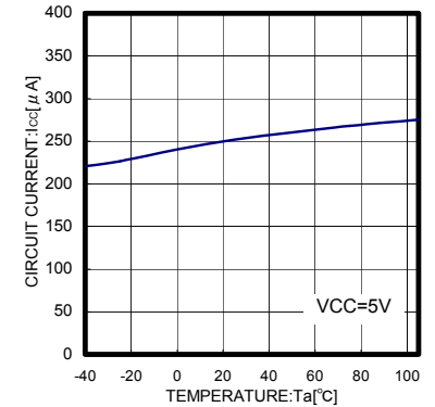
Fig.11 Ta - Icc
