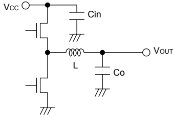
Fig.29 Input capacitor
