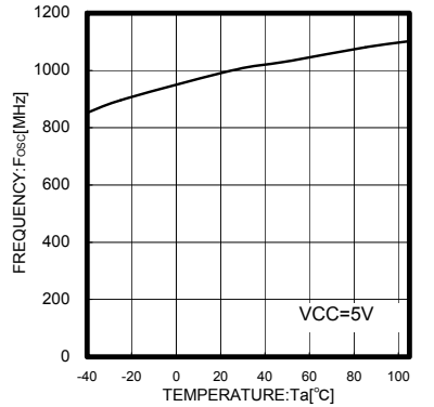
Fig.8 Ta - Fosc
