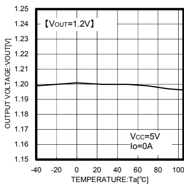
Fig. 6 T a -V OUT
