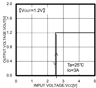
Fig.3 V CC -V OUT
