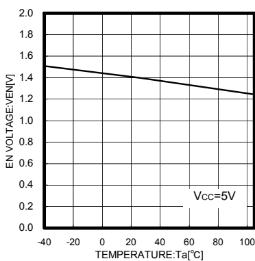
Fig.10 T a -V EN
