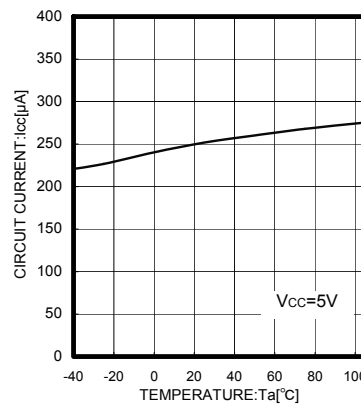
Fig.11 T a -I CC
