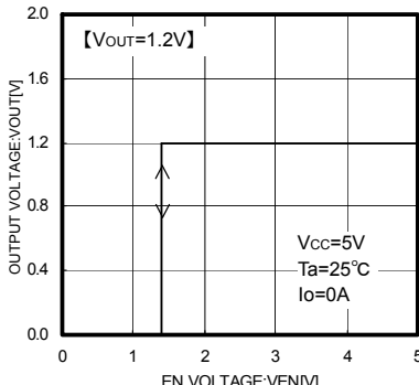
Fig.4 V EN -V OUT
