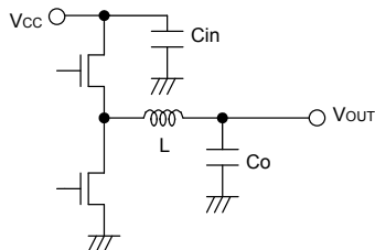
Fig.32 Input capacitor
