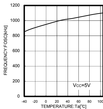
Fig.8 T a -F OSC
