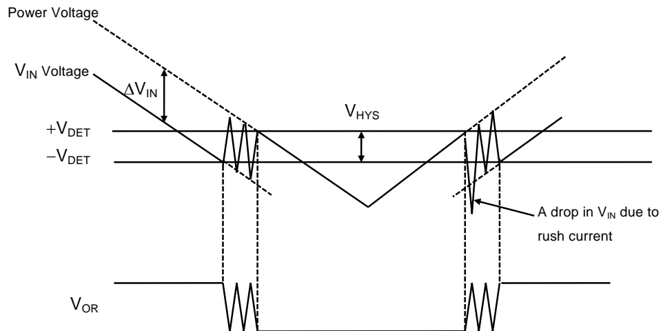
Figure 25 When \Delta V_{IN} > V_{HYS}
