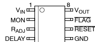
SO-8
