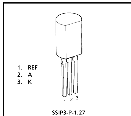
Weight : 0.36 g (Typ.)
