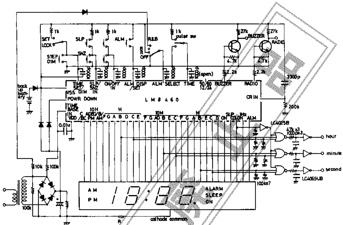
応用回路例2. LED表示用, けた上げ出力つき/12時表示, 60Hz.
