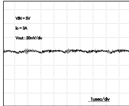
Fig.12 Output ripple
