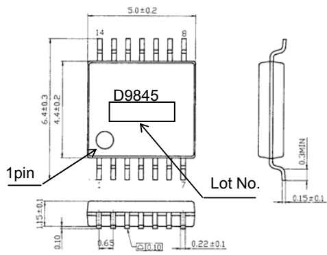
SSOP-B14 [単位:mm]
