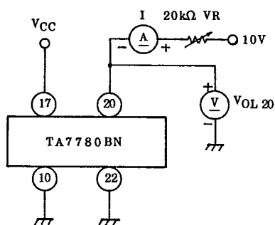
TEST CIRCUIT 9 : VOL20
