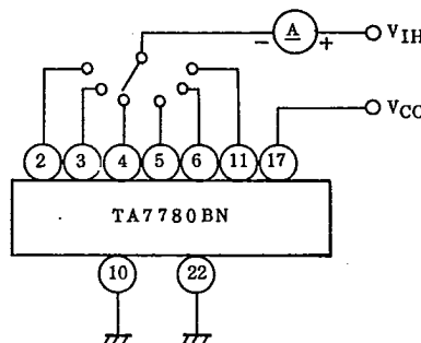
TEST CIRCUIT 2 : I_{IH}
