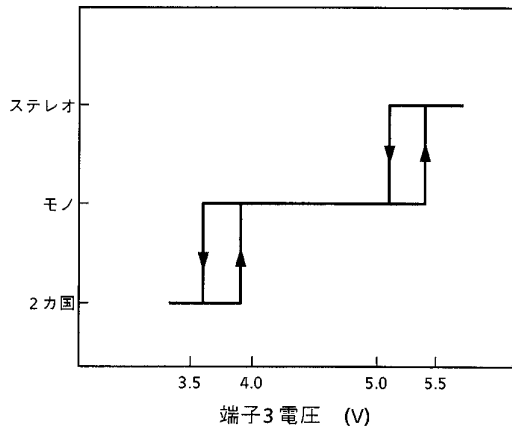
Q信号判別ヒステリシス特性
