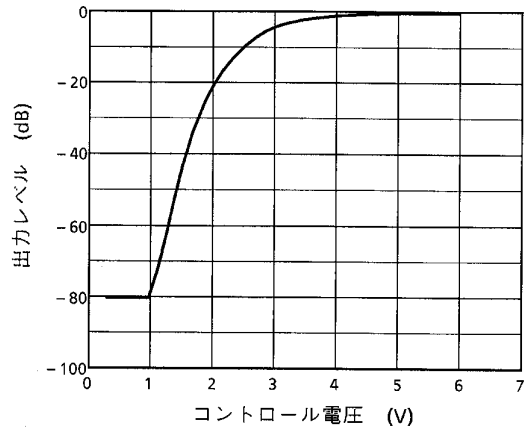
ボリュームコントロール特性
