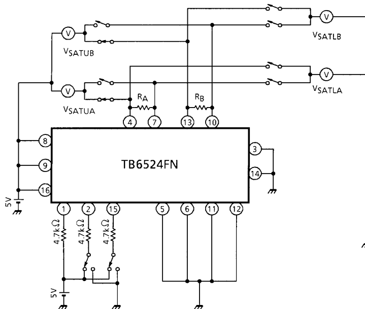
TEST CIRCUIT 3 V_{SAT\ U-1,2} / V_{SAT\ L-1,2}
