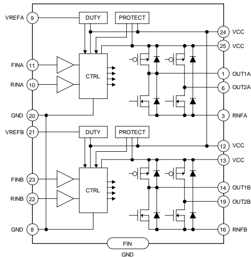
Fig. 33 BD6225FP, BD6226FP
