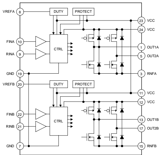
Fig. 31 BD6225FV
