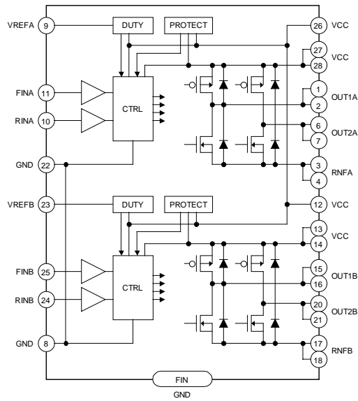
Fig. 36 BD6227FM
