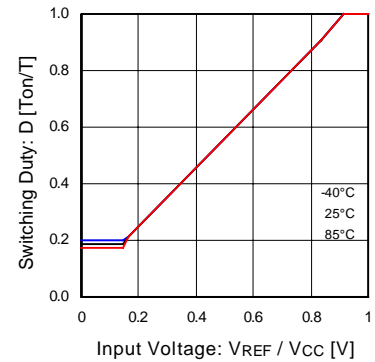
Fig.6 VREF - DUTY (V CC =12V)
