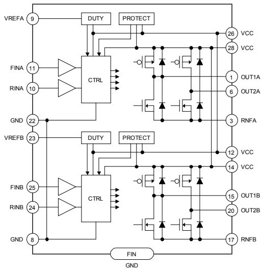
Fig.33 BD6226FM
