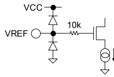
Fig.47 VREF
