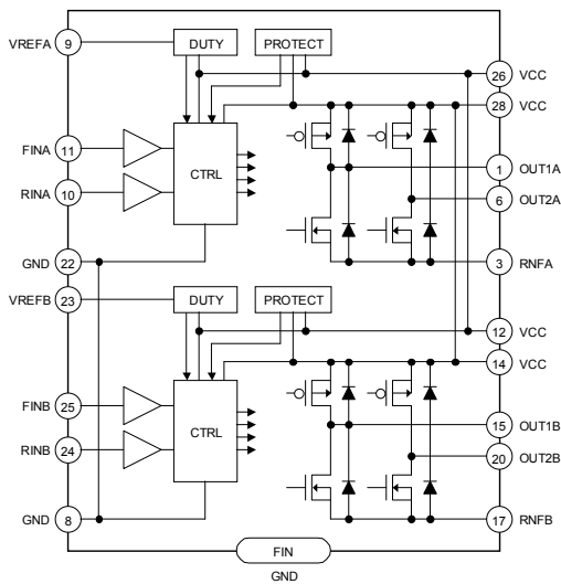
Fig.33 BD6236FM
