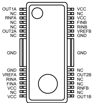
Fig.34 HSOP-M28
