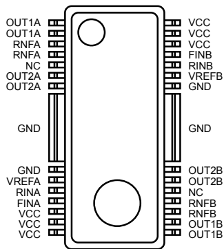
Fig.36 HSOP-M28
