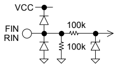
Fig.46 FIN / RIN
