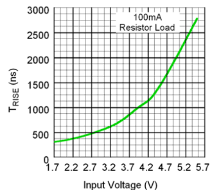
MIC94080/1/2/3/4/5
