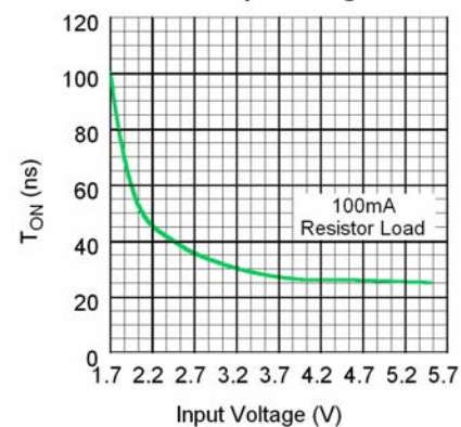
MIC94080/1/2/3/4/5
