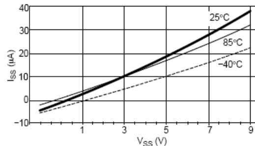
Figure 14. I_{SS} vs. V_{SS}
