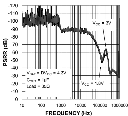
LDO PSRR
