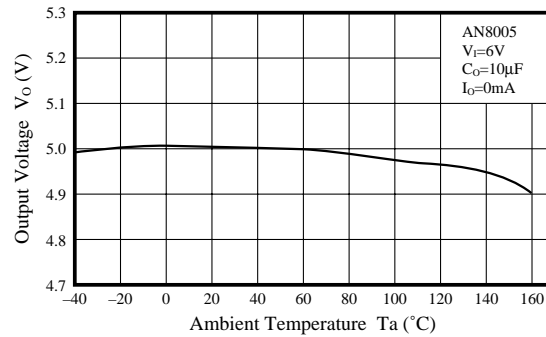
V_O - T_a
