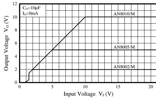
V_O - V_I
