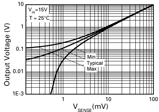
Error v Sense Voltage
