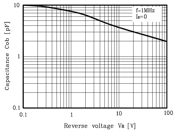
Fig. 4 C_{ob} - V_R
