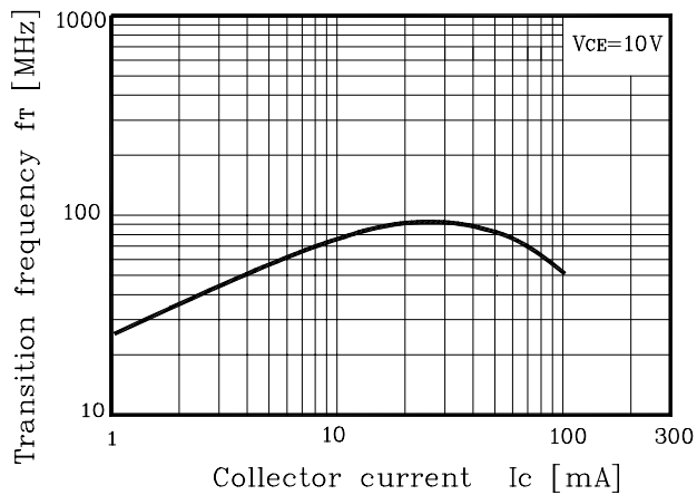
Fig. 3 f_T - I_C
