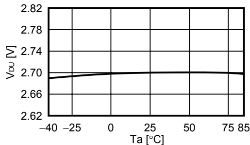
(5) V_{DU} - T_a
