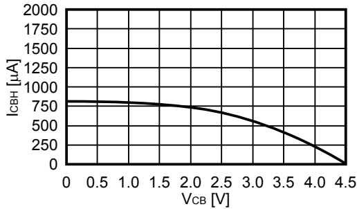
(3) I_{CBH} - V_{CB} ( V_{DS} = 4.5 V)
