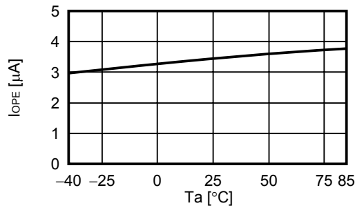
(1) I_{OPE} - T_a
