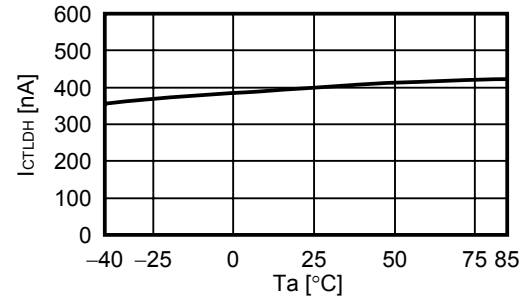
(2) I_{CTLDH} - T_a ( V_{DS} = 3.5 V)
