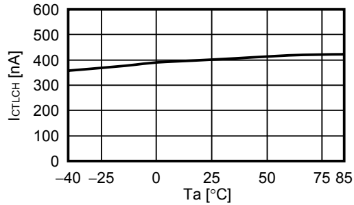
(1) I_{CTLCH} - T_a ( V_{DS} = 3.5 V)
