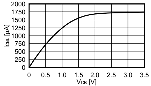
(4) I_{CBL} - V_{CB} ( V_{DS} = 3.5 V)
