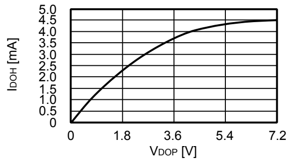
4.3 I_{DOH} vs. V_{DOP}
