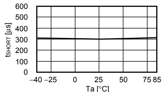
3.8 t_{SHORT}-T_a
